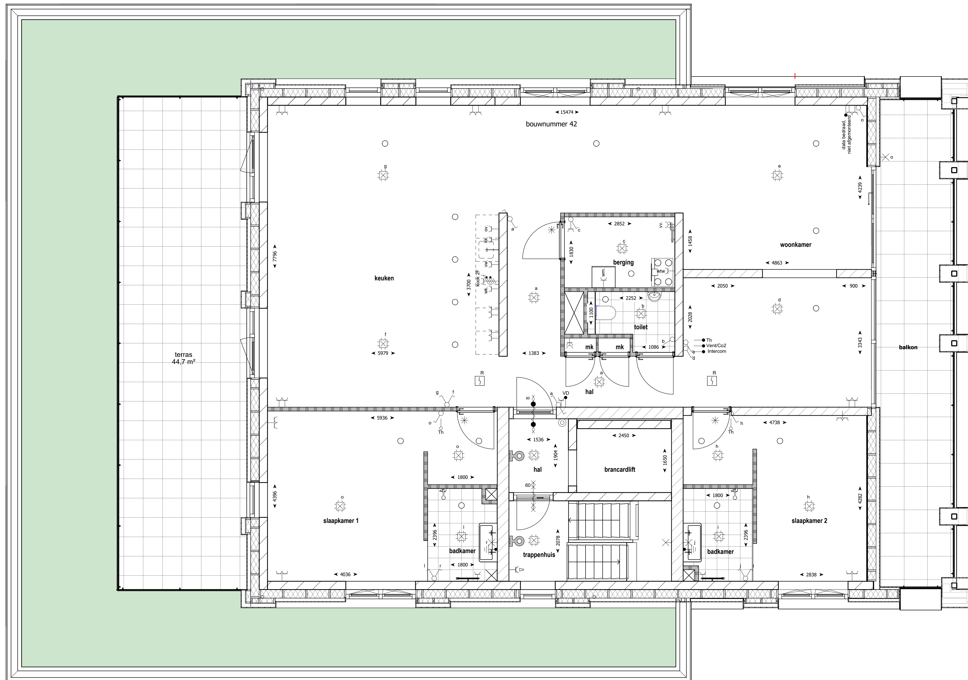
1e verdieping 1 : 50
